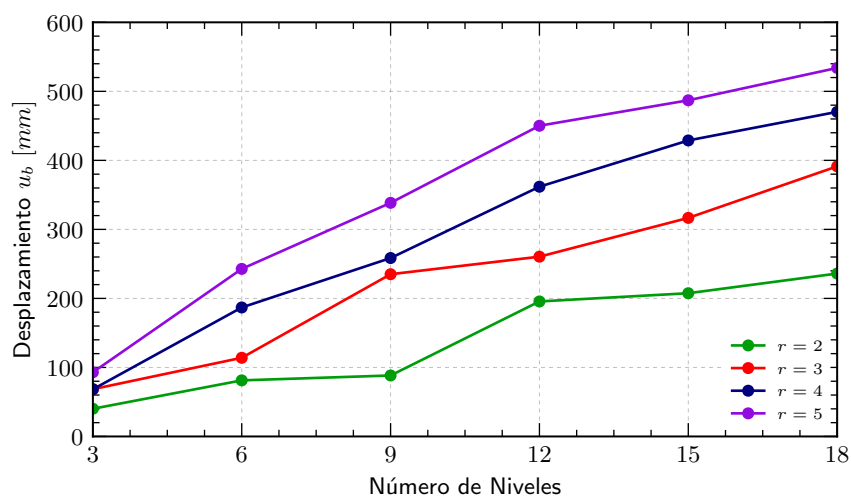
FIGURA N° 3.3: Desplazamiento máximo de la interfaz de aislamiento.
