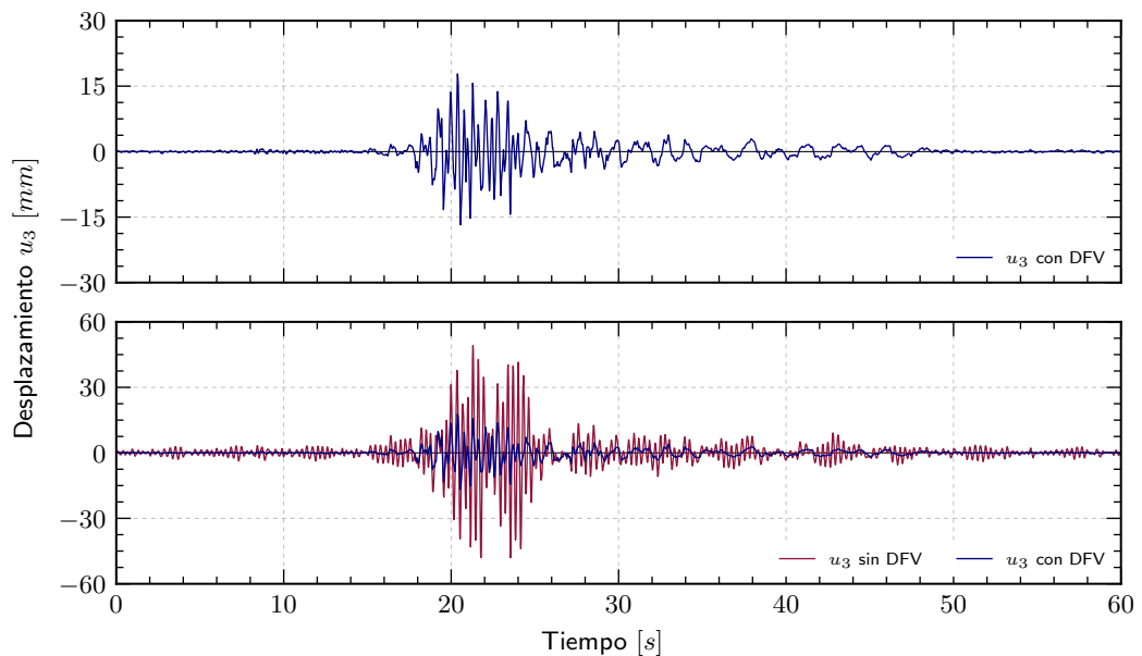
FIGURA N° 4.3: Desplazamiento máximo del último nivel.
