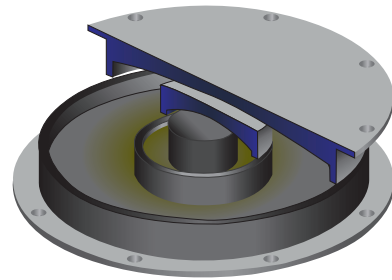
(b) Aislador friccionante TFPB. Adaptado de Fenz y Constantinou (2008)
